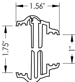
3A OD LITE FRAME HP POLYPROPYLENE
